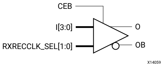
OBUFDS_GTE3_ADV
